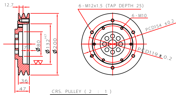
CRS. PULLEY ( 2 : 1 )
